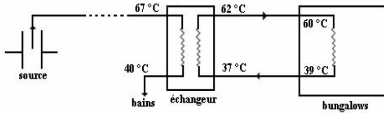
Fig. 3: Schéma du circuit de distribution
