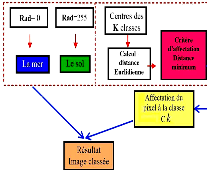
Fig. 4: Les différentes étapes de l'algorithme de classification
