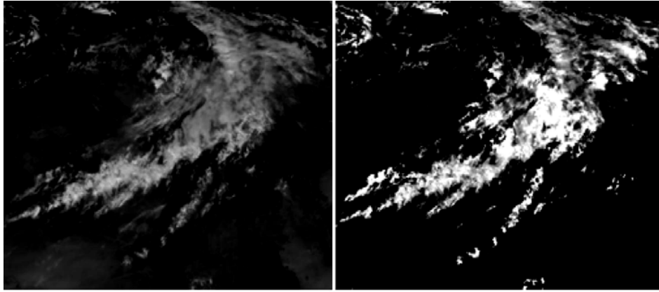
Fig. 3: Données satellitaires utilisées à droite, image ennuagement, à gauche, image visible
