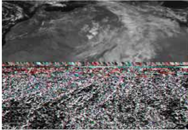
Fig. 5: Image visible à gauche
