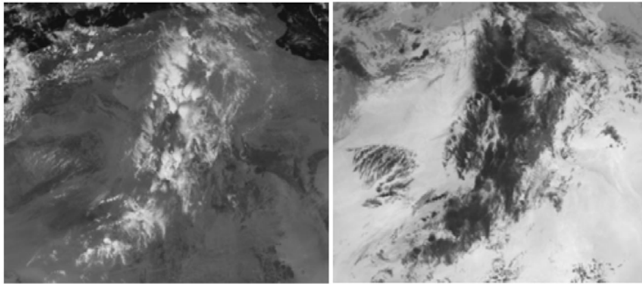
Fig. 1: Données satellitaires utilisées à droite, vue prise dans le canal infrarouge, à gauche, vue prise dans le canal visible (ONM, Algérie)
