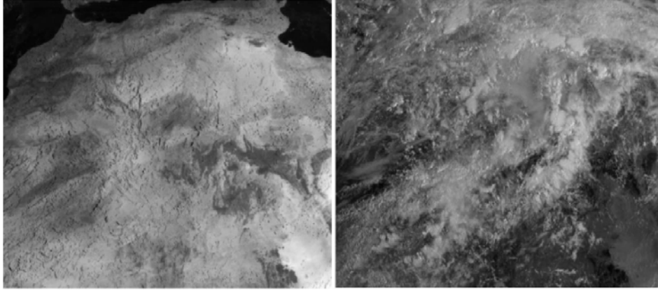
Fig. 1: Données satellitaires utilisées à droite, image prise à ciel couvert, à gauche, image prise à ciel clair
