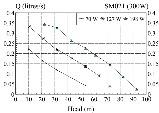
Fig. 5: Débit de la pompe pour une puissance utile P_a=70, 127 et 198 W
