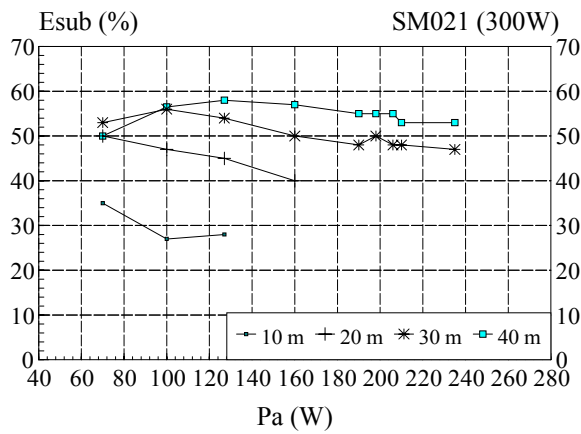
Fig. 8: Rendement de pompage pour hmt=10, 20, 30 et 40 m
