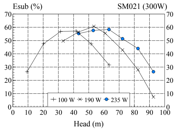
Figure 3: Rendement de pompage pour une puissance utile P_a=100, 190 et 235 W
