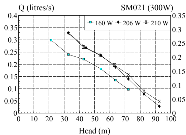
Fig. 7: Débit de la pompe pour une puissance utile P_a = 160, 206 et 210 W
