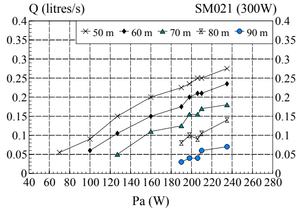
Fig. 11: Débit de la pompe pour hmt = 50, 60, 70, 80 et 90 m
