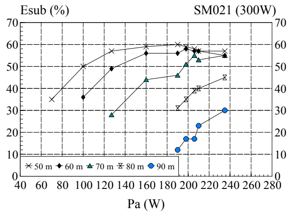
Figure 9: Rendement de pompage pour hmt=50, 60, 70, 80 et 90 m
