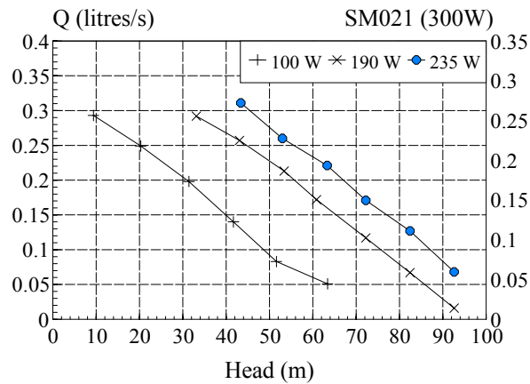
Figure 6: Débit de la pompe pour une puissance utile P_a=100, 190 et 235 W
