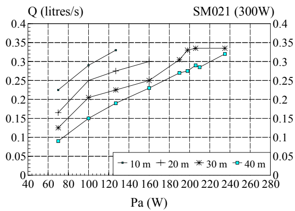
Fig. 10: Débit de la pompe pour hmt = 10, 20, 30 et 40 m
