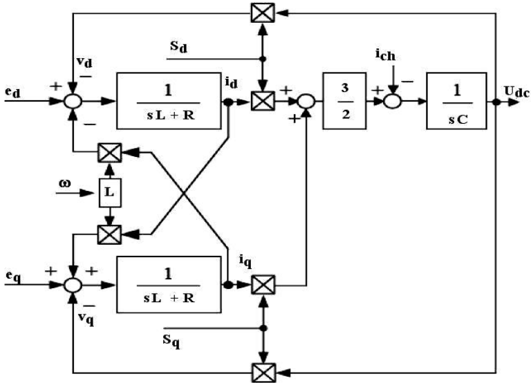
Fig. 7: Schéma fonctionnel du redresseur MLI de tension dans le référentiel tournant d - q
