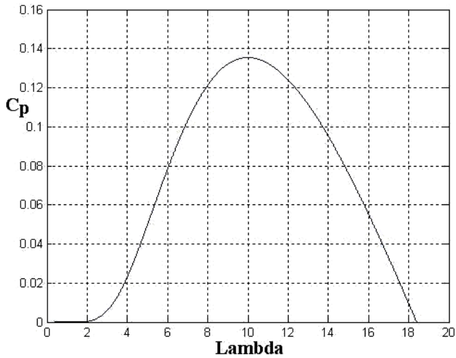
Fig. 2: Coefficient aérodynamique en fonction du ratio de vitesse de la turbine ( \lambda )
