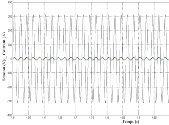
Fig. 11: Variation de la tension et du courant de la GADA (Zoom)
