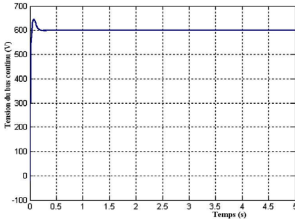
Fig. 12: Variation de la tension redressée en fonction du temps
