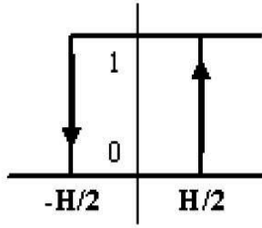
Fig. 6: Principes de fonctionnement de Modulateur MLI à bande d'hystérésis
