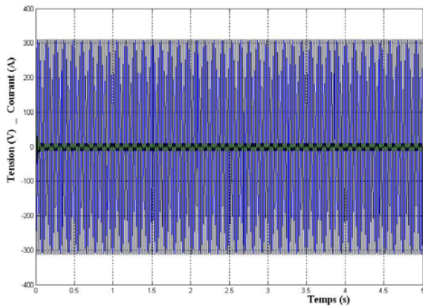
Fig. 10: Variation de la tension et du courant de la GADA
