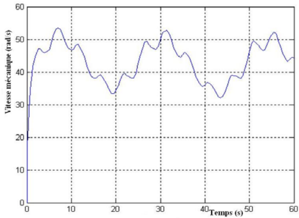
Fig. 9: Variation de la vitesse mécanique (rad/s)
