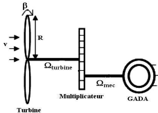
Fig. 3: Structure du système de conversion éolien
