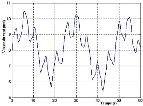
Fig. 8: Variation de la vitesse du vent (m/s)
