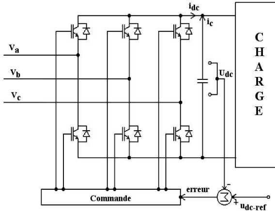
Fig. 5: Topologies de base d'un redresseur de tension
