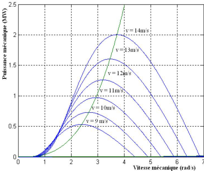
Fig. 4: Puissance théorique disponible pour un type d'éolienne donnée
