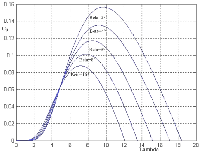
Fig. 1: Coefficient de puissance en fonction du ratio de vitesse ( \lambda ) et de l'angle de calage ( \beta )
