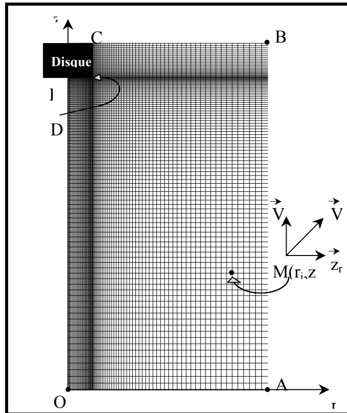
Fig. 4 : Maillage du domaine de calcul \overline{OABCE} comportant 83 \times 109 nœuds respectivement selon les axes or et oz. (OA=150mm, AB=300mm, BC=130.25mm, CD=30mm, DE= R_D =19.75mm, EO=270mm)
