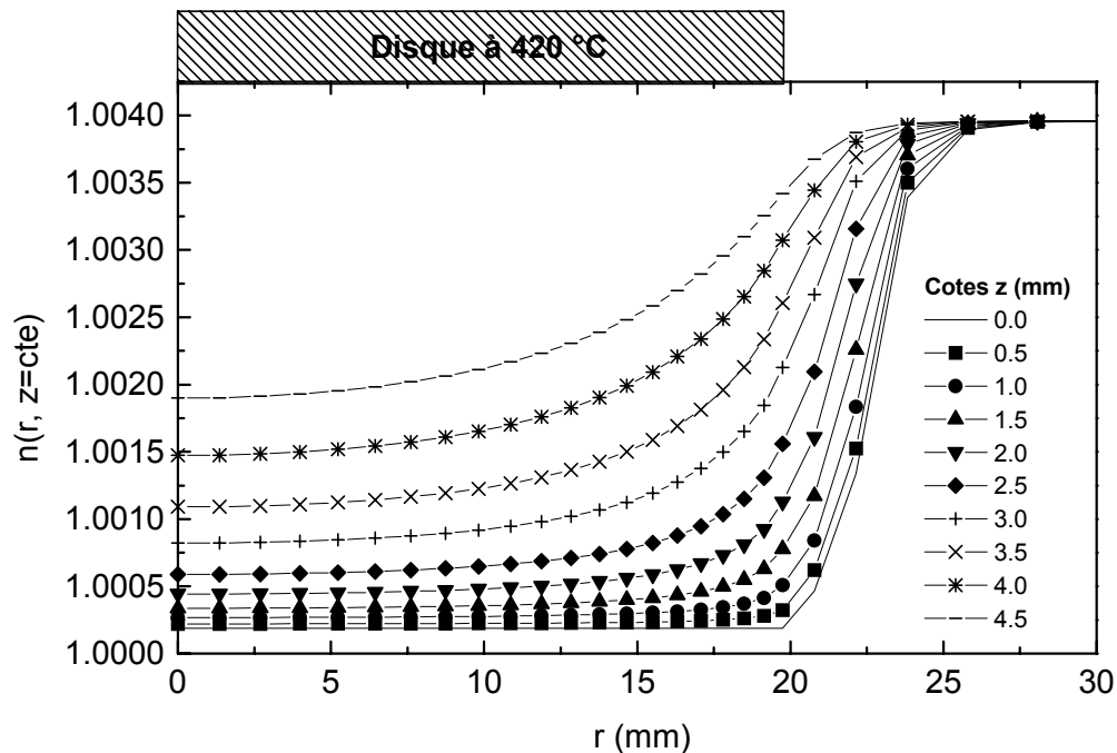
Fig. 10 : Distribution radiale de l'indice de réfraction sous le disque pour plusieurs cotes ( z = \text{cte} )
