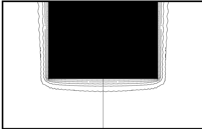
Fig. 6 : Les isothermes autour du disque à 420°C de 40 à 400°C avec un pas de 80 °C
